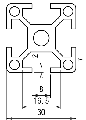
適合アルミフレーム寸法
