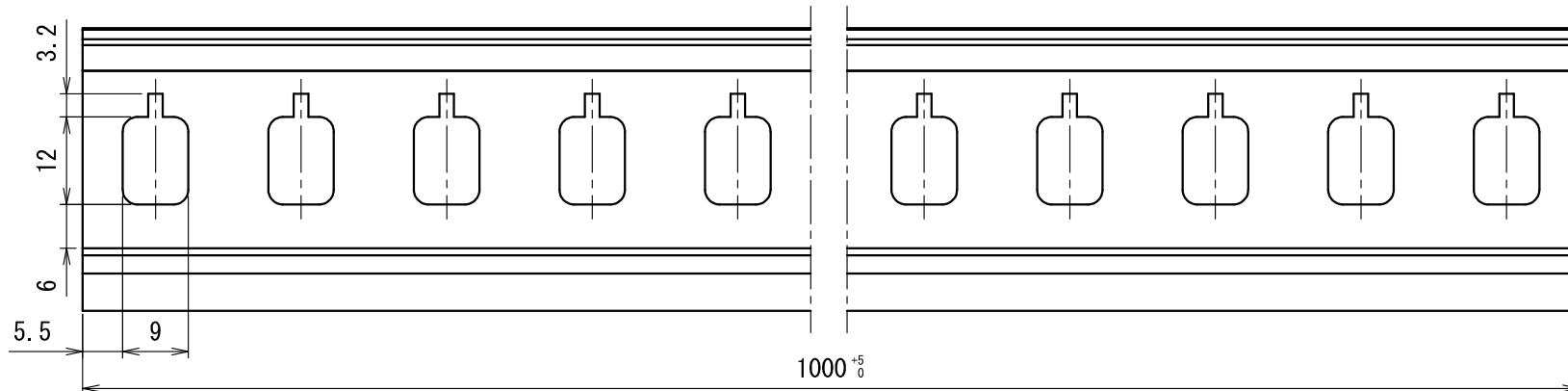
適合アルミフレーム寸法
