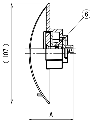
断面 A-A
