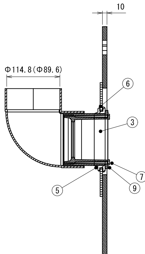
断面 A-A
