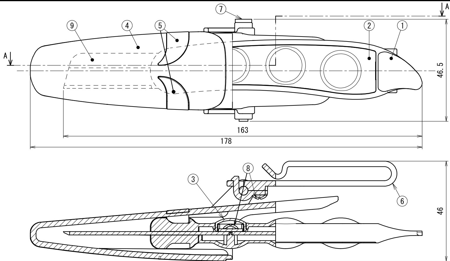
断面 A-A
