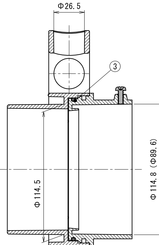
断面 A-A
