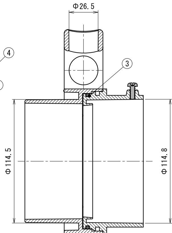
断面 A-A
