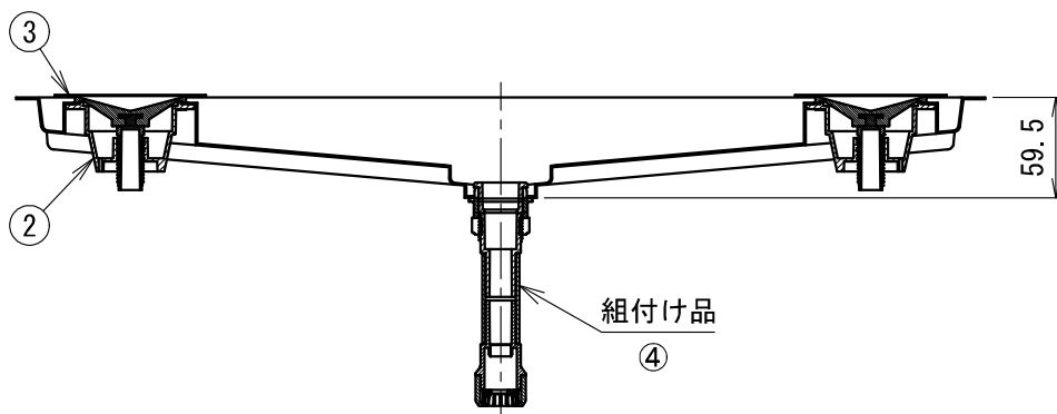
断面 A-A
