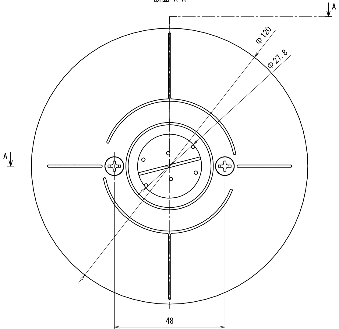
断面 A-A
