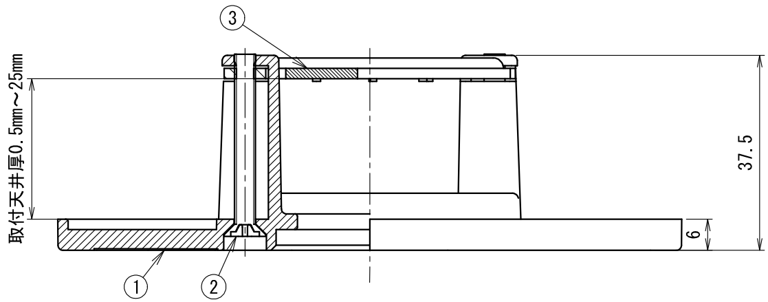
断面 A-A
