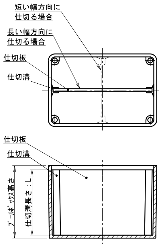
仕切板取り付け状態
