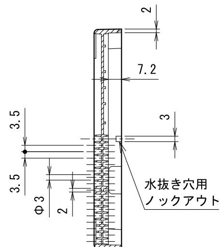
A-A断面図
