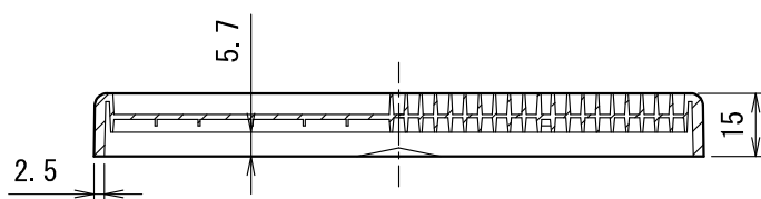
A-A断面図
