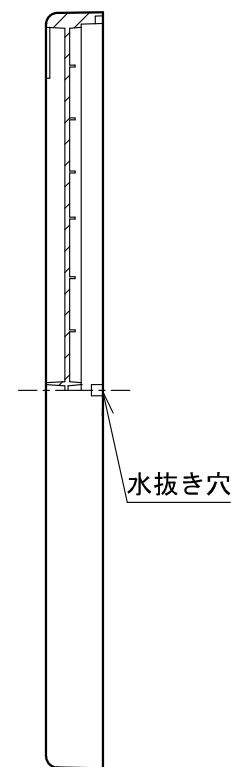
B-B断面図
