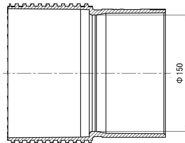
断面 A-A
