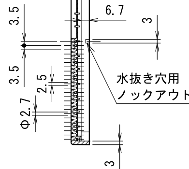
A-A断面図
