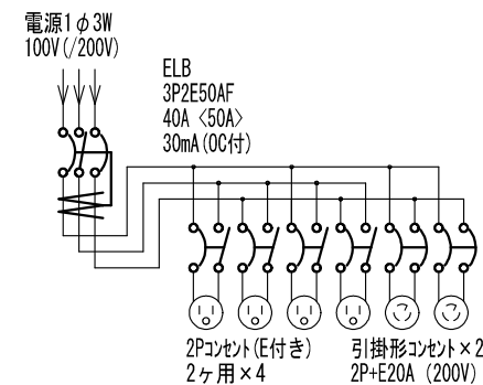
結線図
