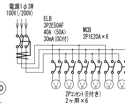
結線図
