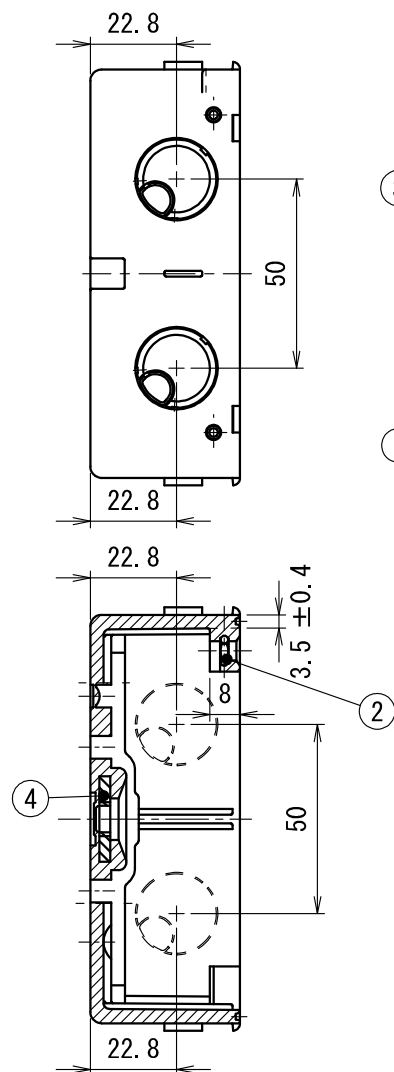
A-A 断面図
