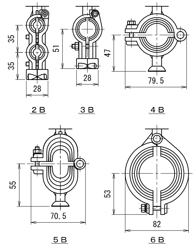
ブラケット
