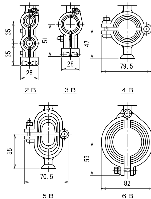
ブラケット
