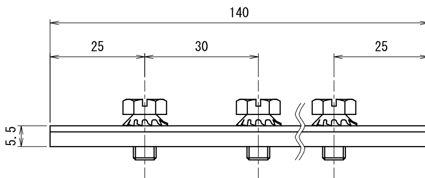
上部連結金具
