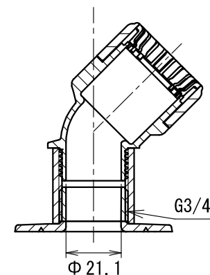
断面 B-B
