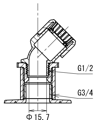
断面 A-A
