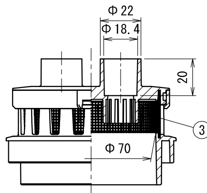
断面 A-A
