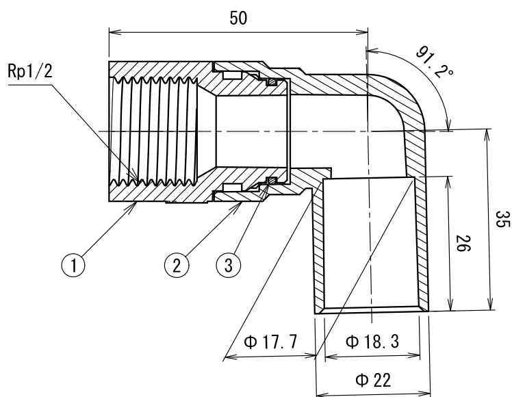
A-A 断面図
