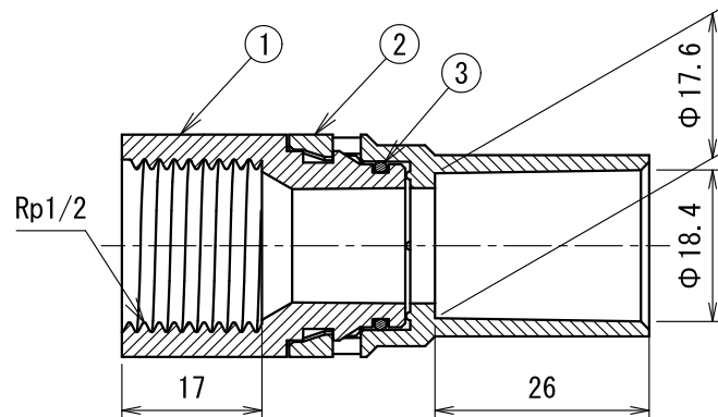
A-A 断面図
