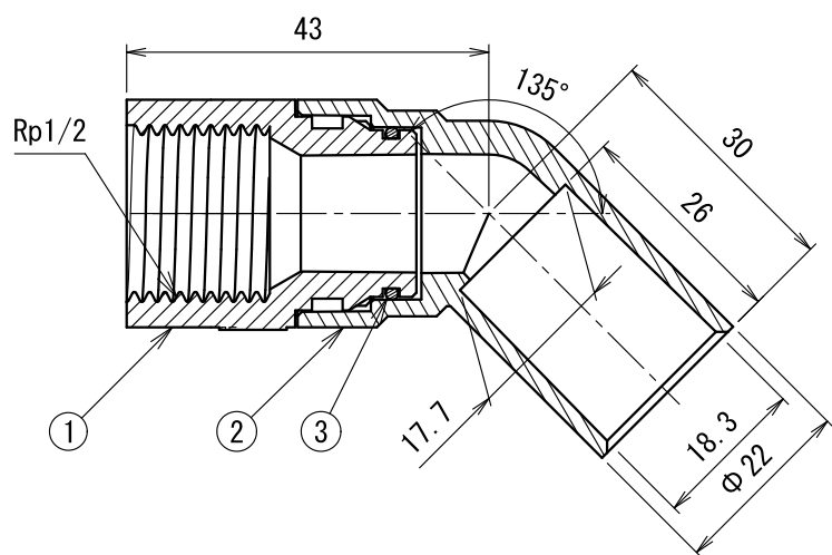
A-A 断面図
