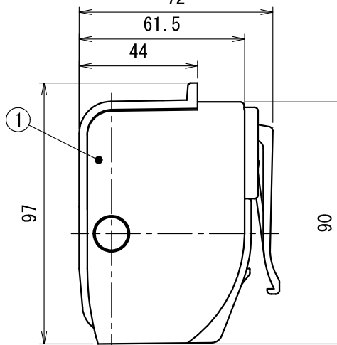
断面 A-A 72
