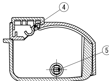
断面 A-A 72
