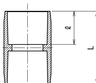
断面 A-A
