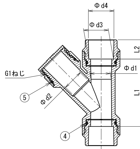
断面 A-A
