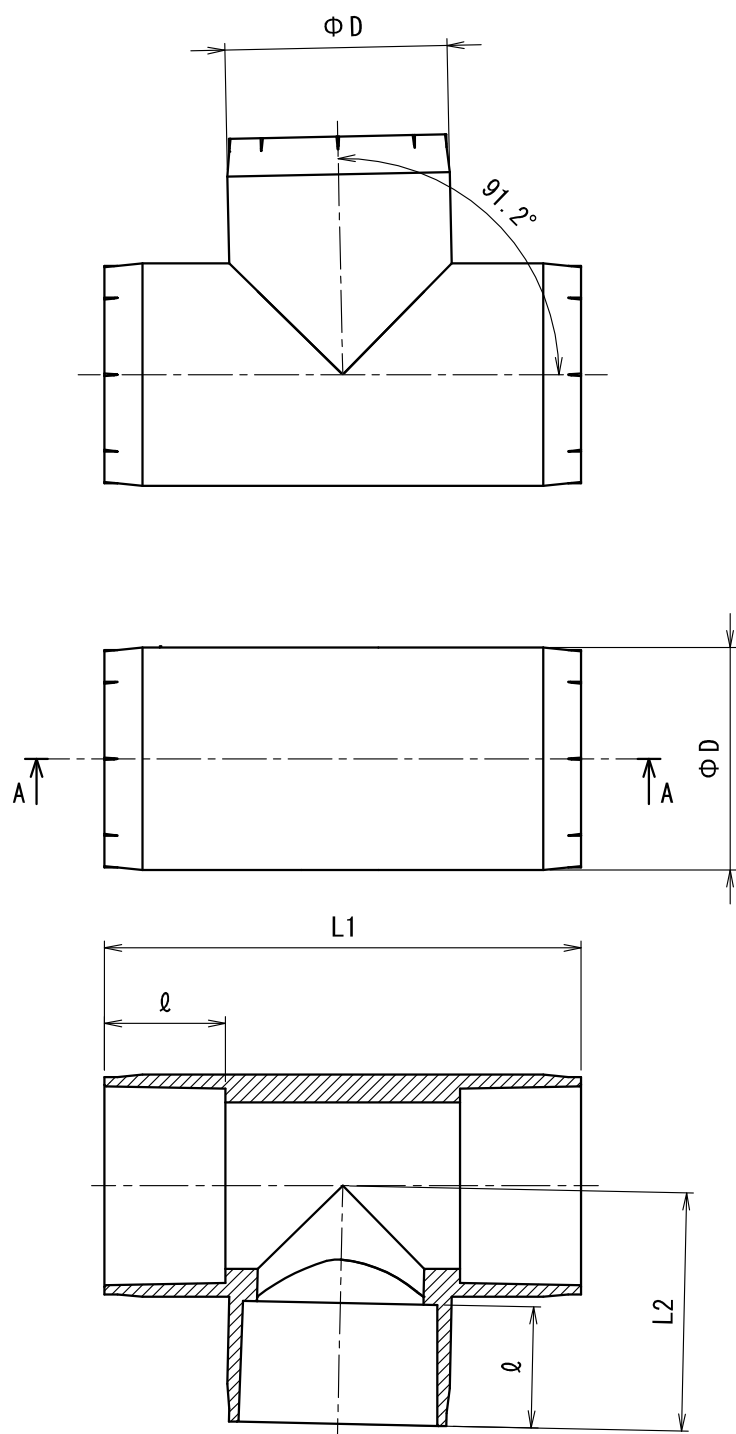
断面 A-A
