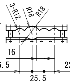
ブッシュEH
