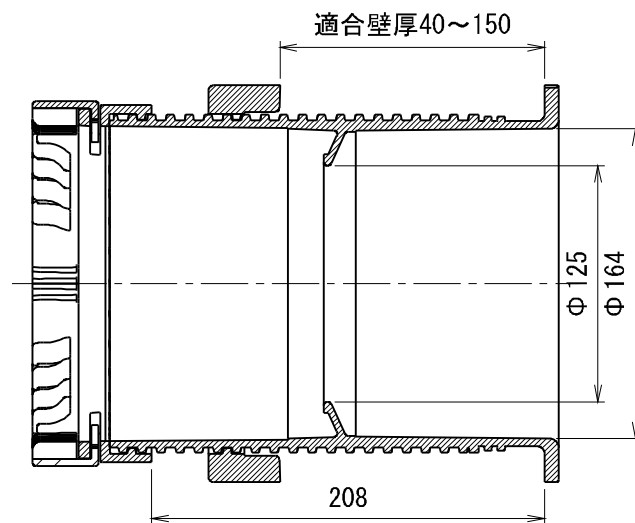
断面 A-A
