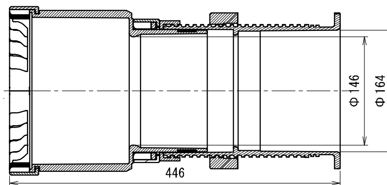
断面 A-A (組付状態)
