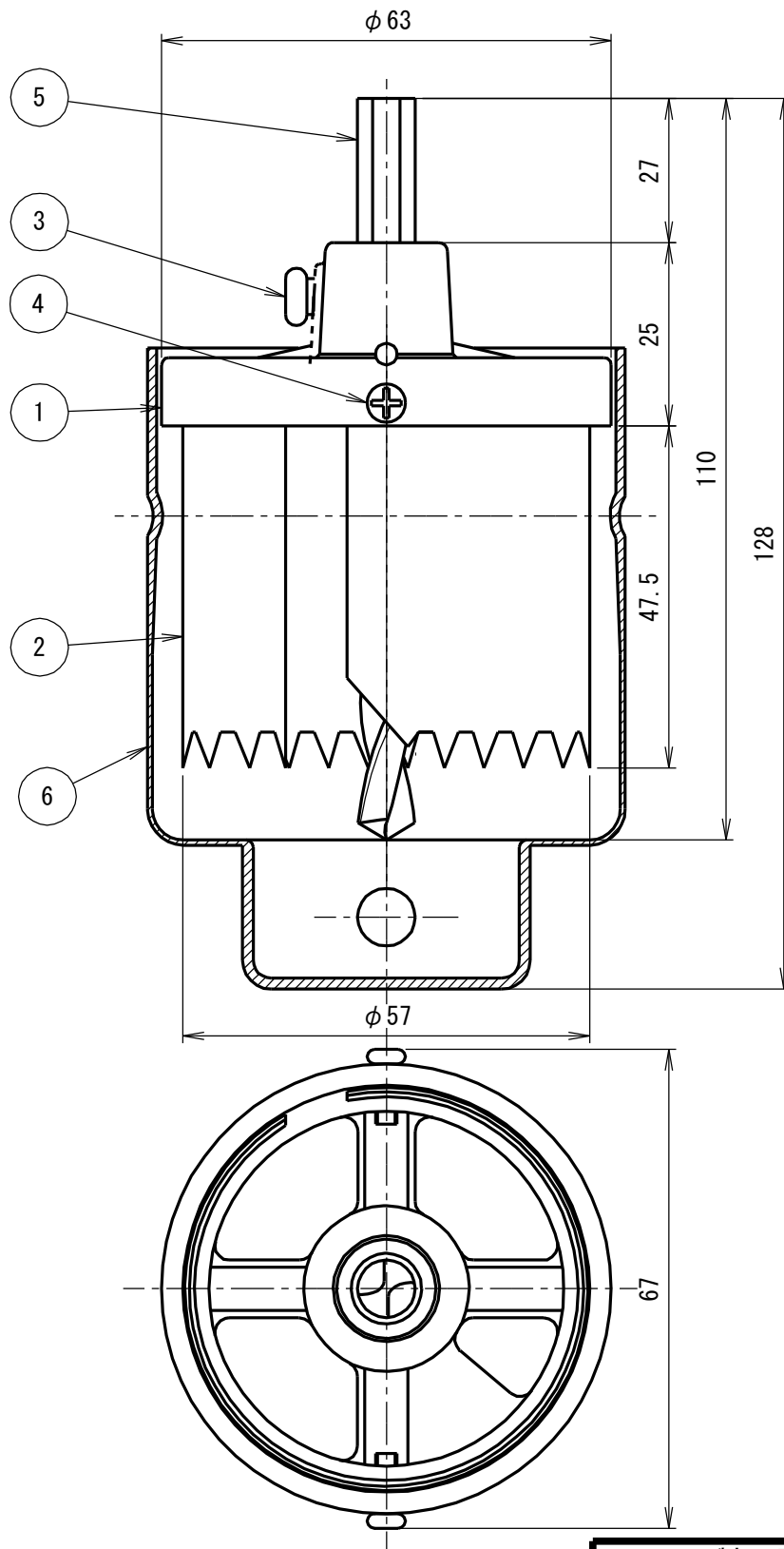
製品仕様図
