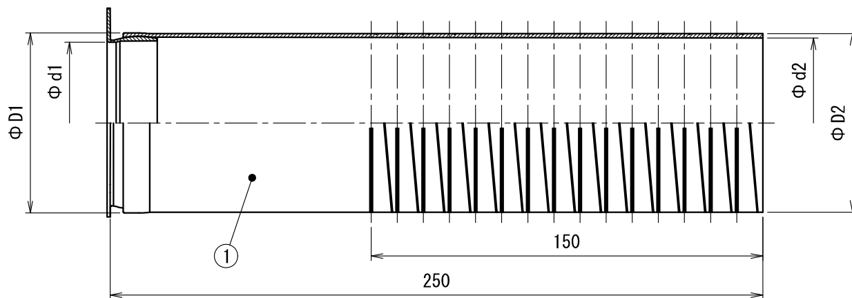
断面 A-A
