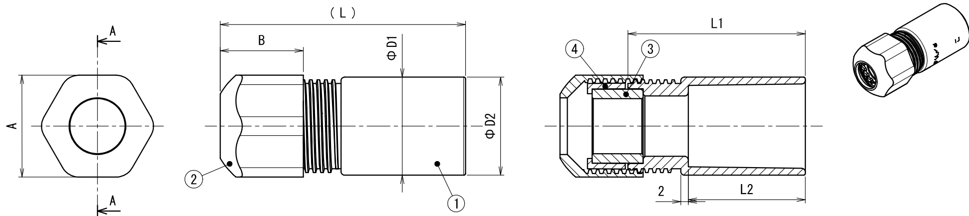
断面 A-A
