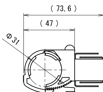
取付最大径
