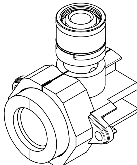
参考斜視図
