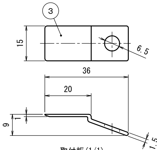
取付板 (1/1)
