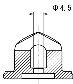
断面 A-A
