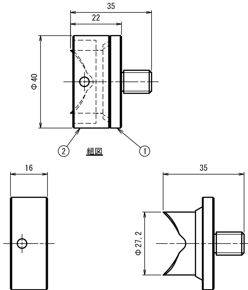
ダイ Φ28
