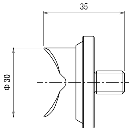
パンチ Φ30
