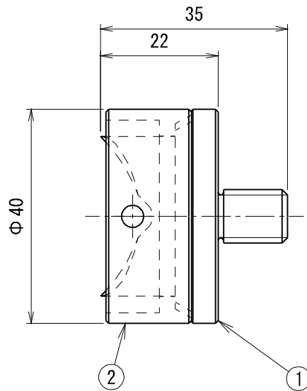
組図
