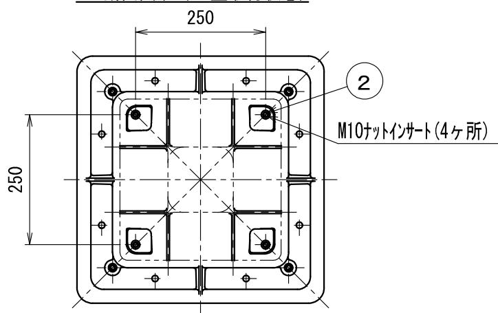
X-X断面図(マンホール蓋取付状態)
