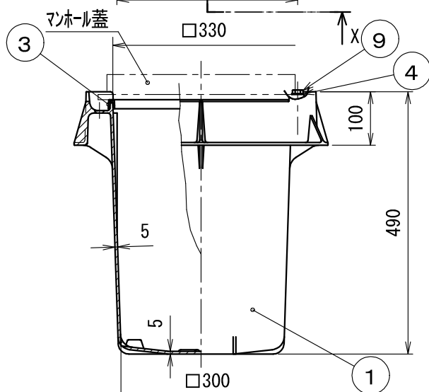
X-X断面図(マンホール蓋取付状態)
