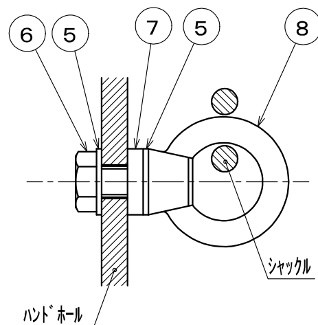
アイボルト固定状態(1/1)
