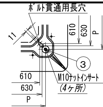
MH-600、6090 ナットインサート部詳細
