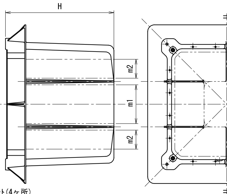
MH-600、6090 ナットインサート部詳細
