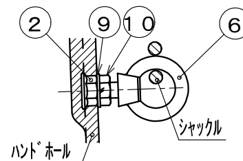
Y-Y断面図(アイボルト固定状態) (1/2)
