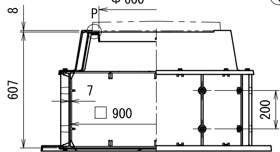
断面 A-A(マンホール蓋取付状態)
