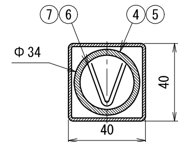
角パイプ断面図 (1/2)
