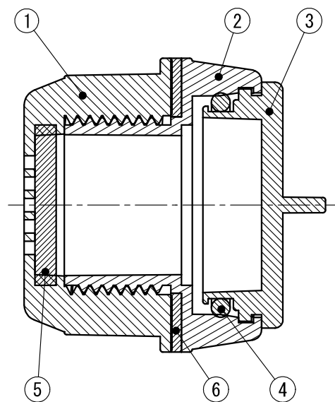
断面 A-A
