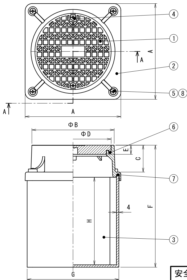
断面 A-A
