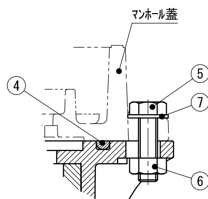
P部詳細図 (1/2) マンホール蓋固定状態
