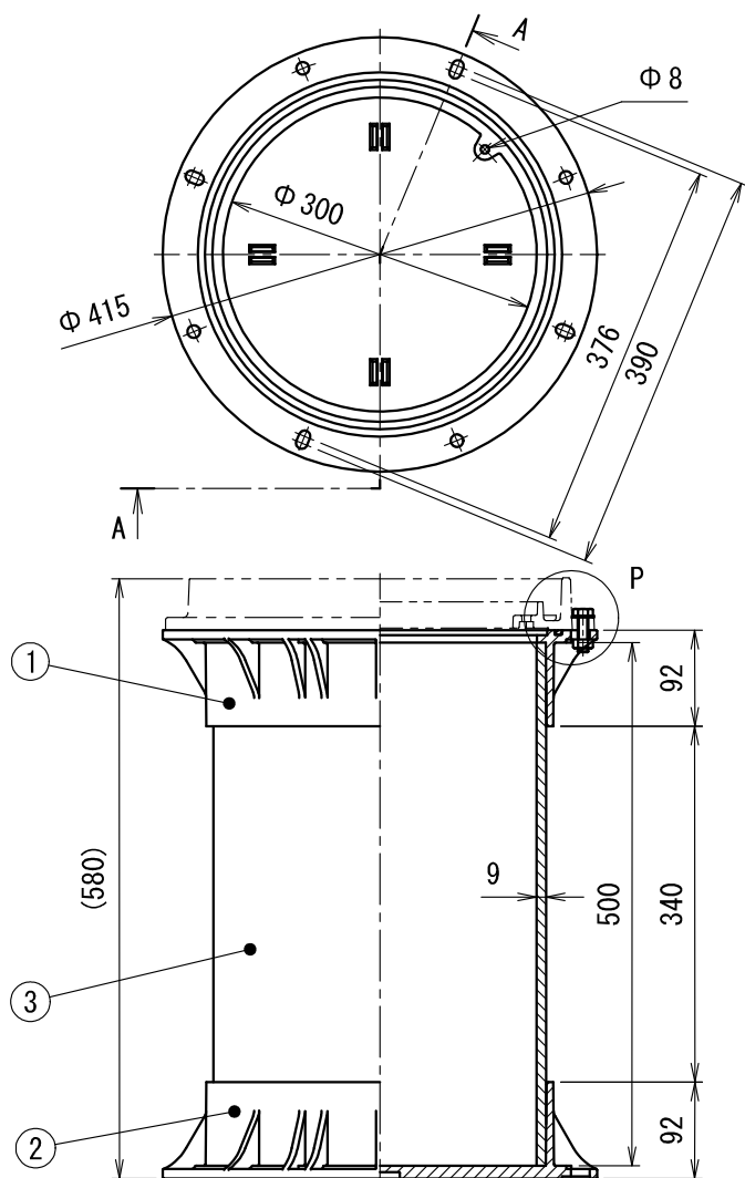
A-A断面図 マンホール蓋 (MKPBR-300) 取付状態
