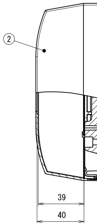
ノック 上下 1号・2号・3号モール
