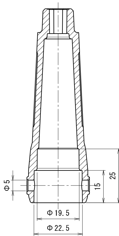
断面 A-A
