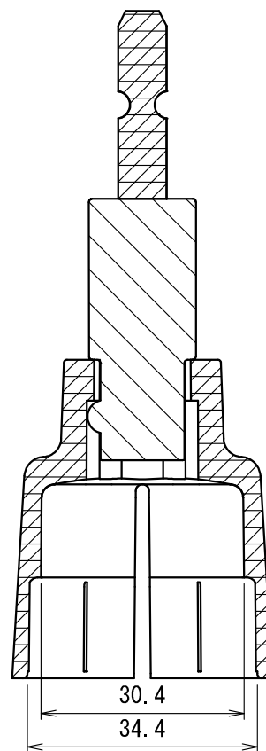
A-A 断面図
